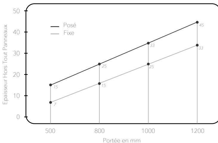
Graphique de dimensionnement pour une charge de 250 Kg/m 2
